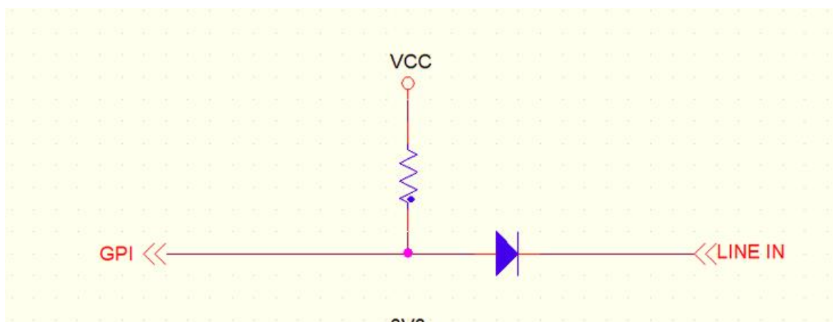
设备输入电路图
