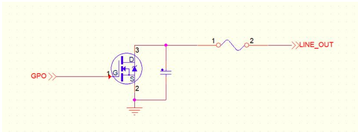
设备输出电路图
