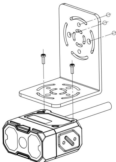
演示图：正面安装
