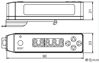
显示盒尺寸
