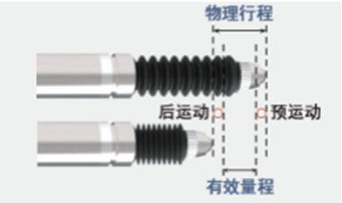
传感器行程尺寸示意
