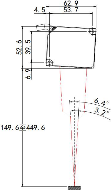
镜面反射型的安装
