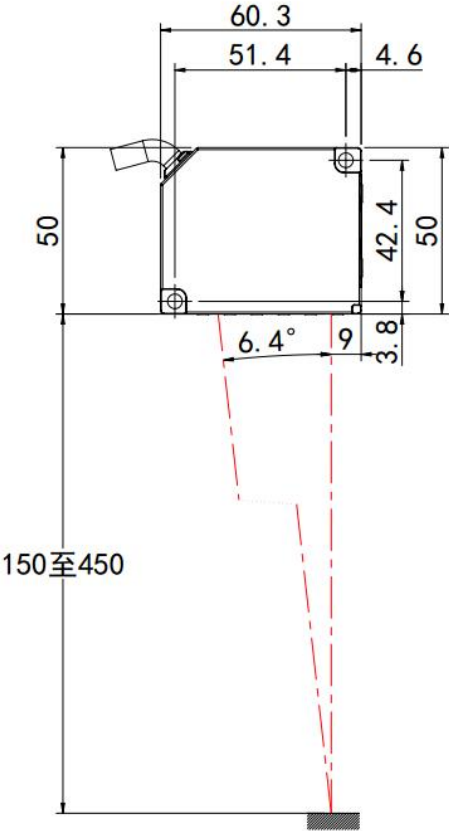
漫反射型的安装
