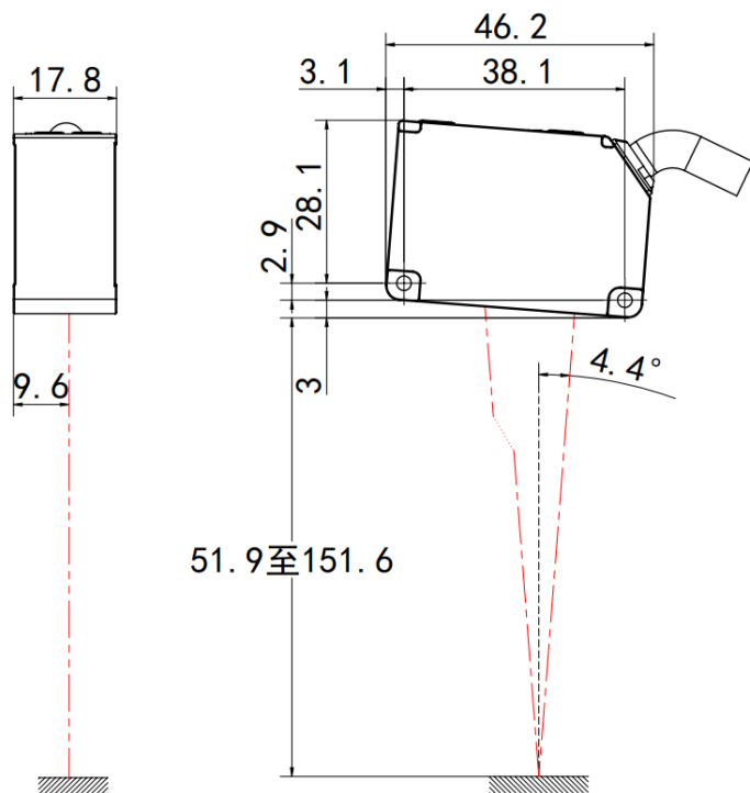
镜面反射型的安装
