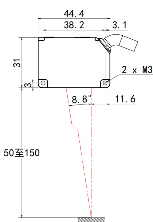
漫反射型的安装
