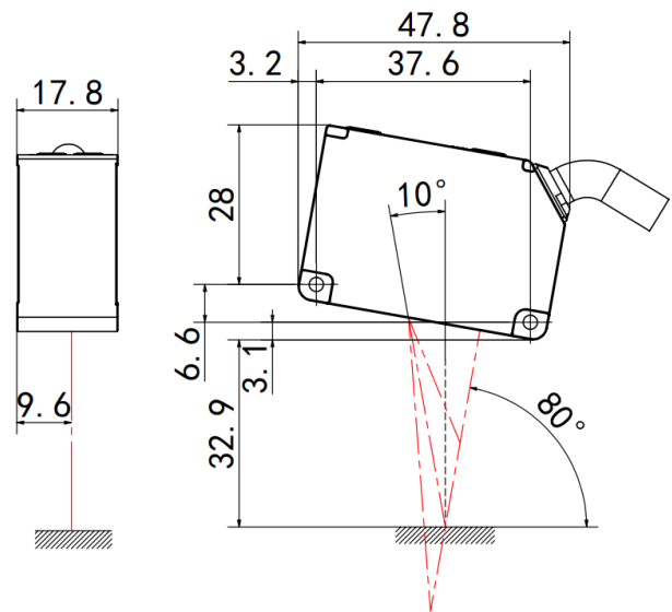
镜面反射型的安装
