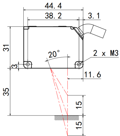
漫反射型的安装
