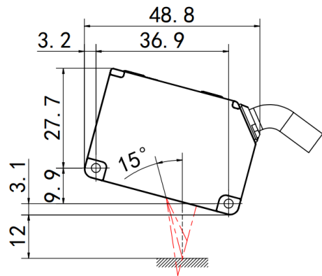
镜面反射型的安装
