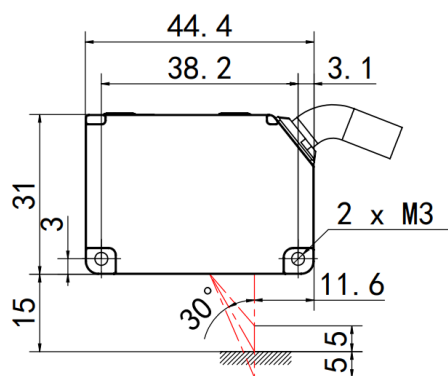
漫反射型的安装
