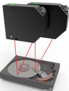
测量HDD的跳动
