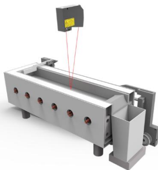
测量回流焊浸 焊槽的液位
