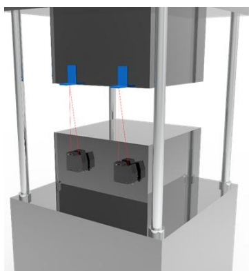
冲压的冲程测量
