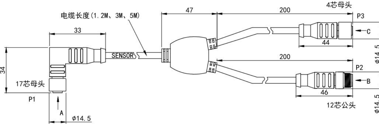
GLX-CCJY2L，弯头电缆尺寸图
